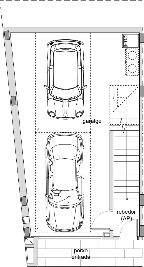
PLANTA BAIXA
