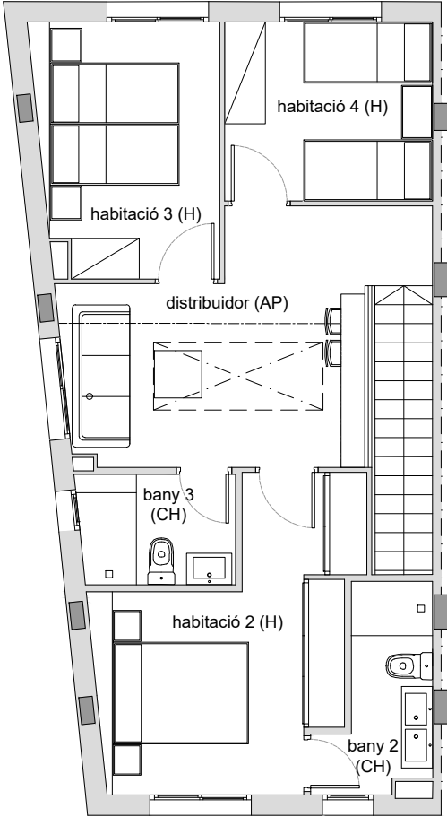
PLANTA SEGONA
