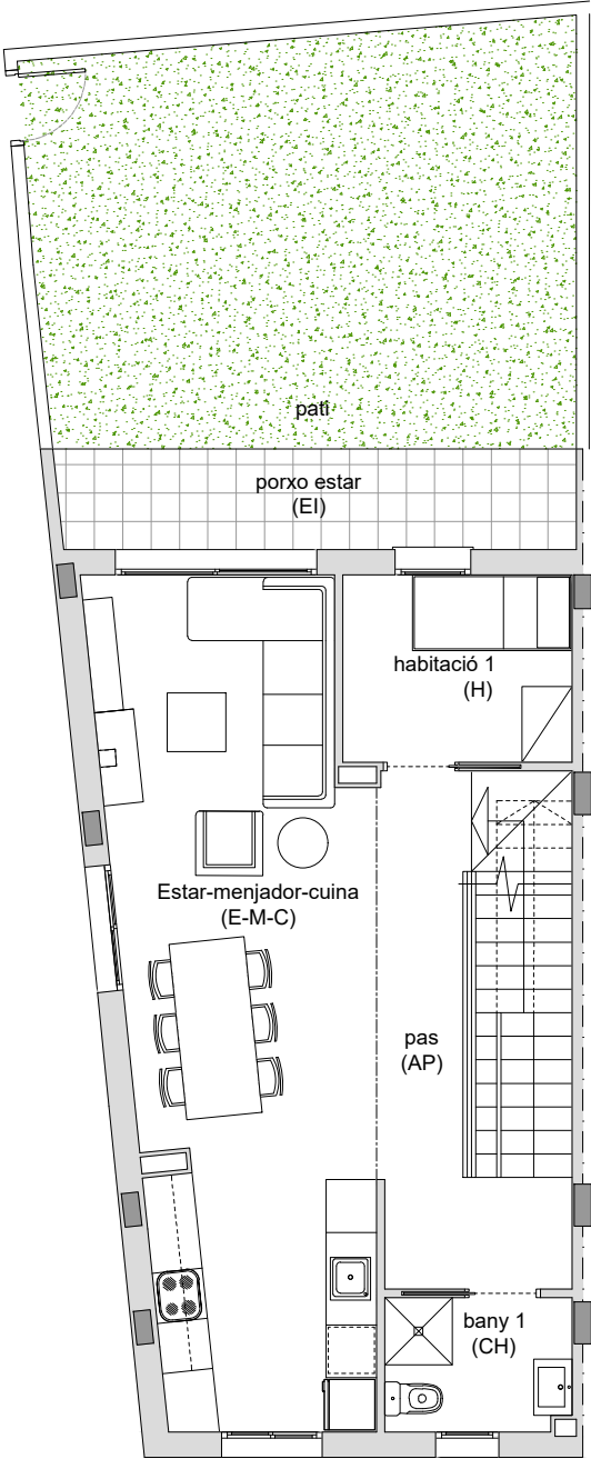
PLANTA PRIMERA
