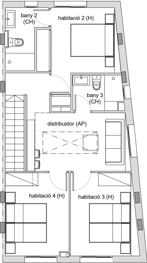
PLANTA SEGONA
