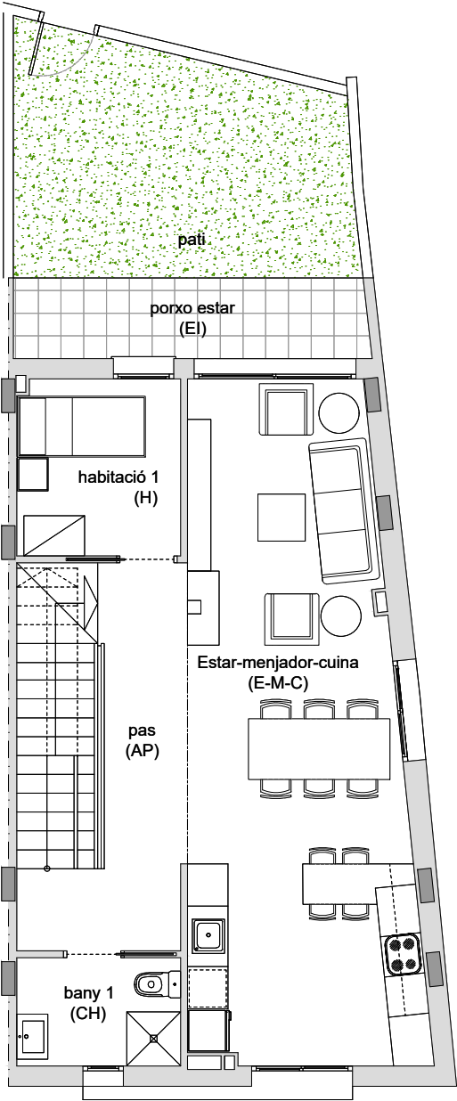
PLANTA PRIMERA
