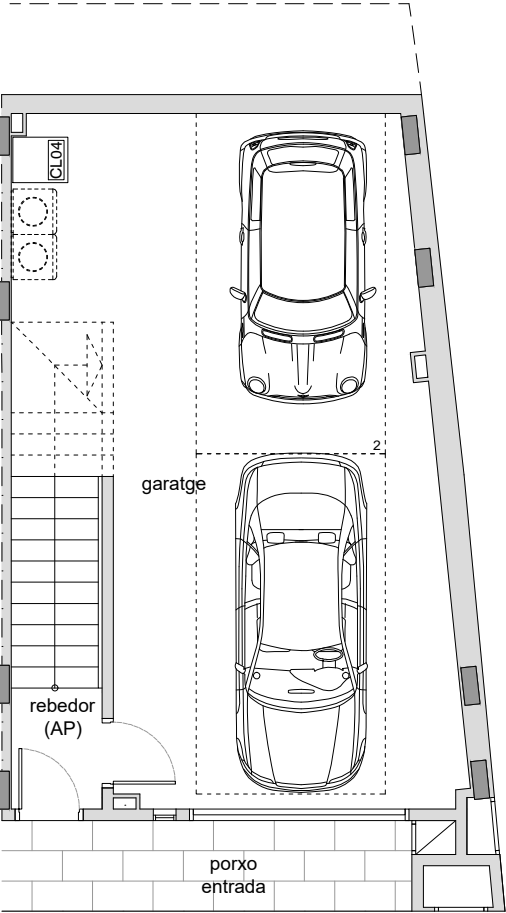
PLANTA BAIXA
