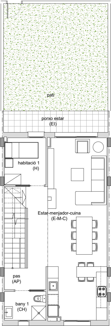
PLANTA PRIMERA
