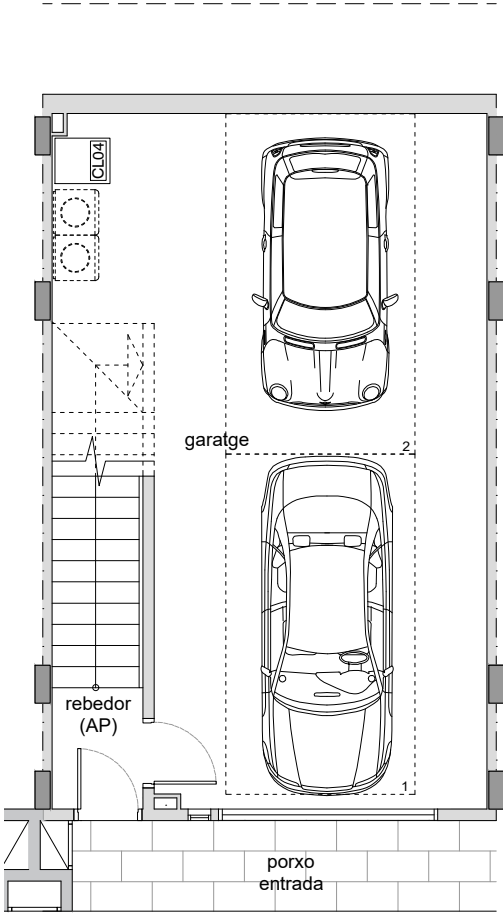
PLANTA BAIXA
