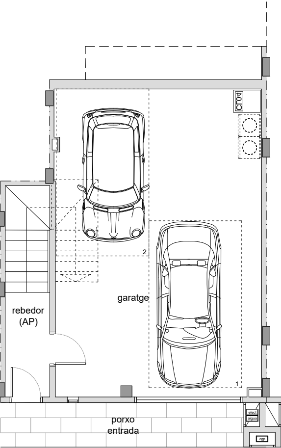
PLANTA BAIXA
