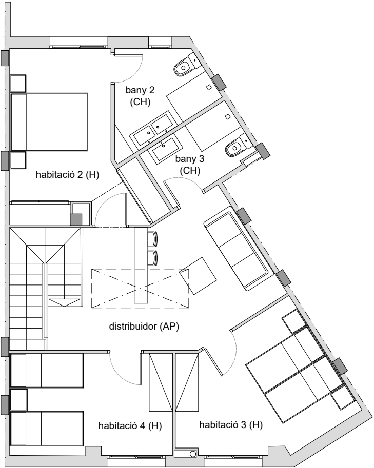
PLANTA SEGONA
