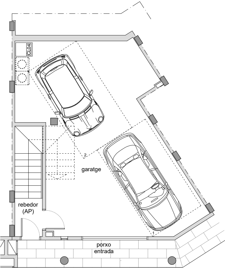
PLANTA BAIXA
