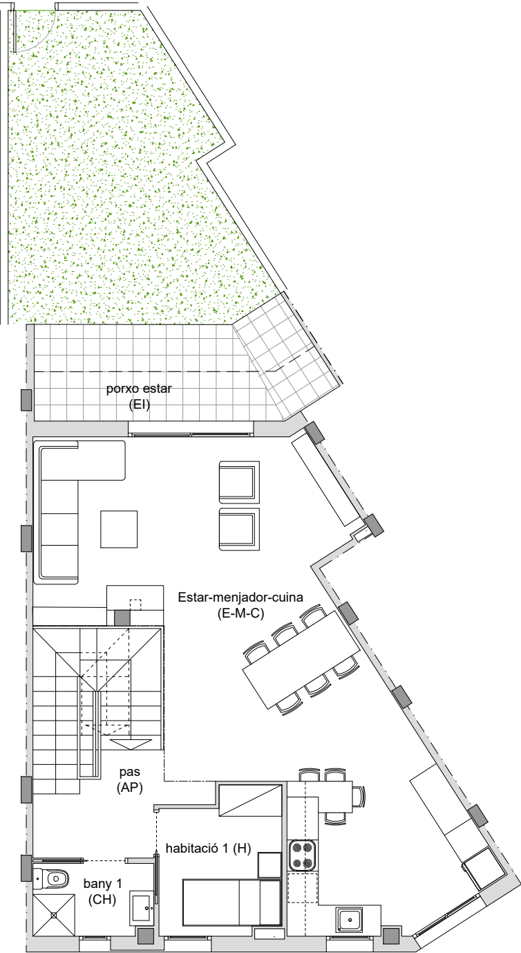
PLANTA PRIMERA
