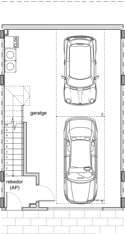
PLANTA BAIXA
