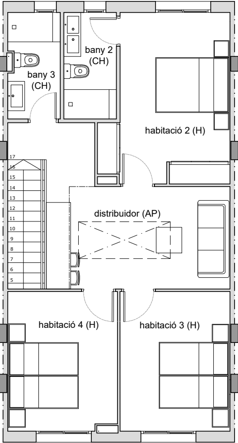
PLANTA SEGONA
