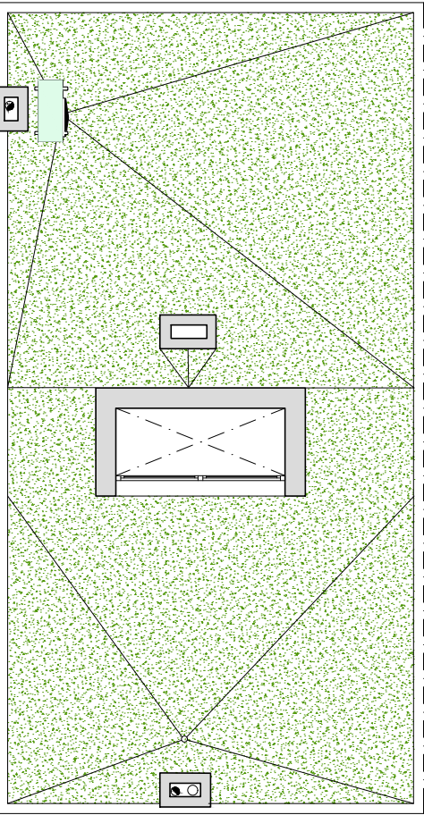
PLANTA COBERTA
